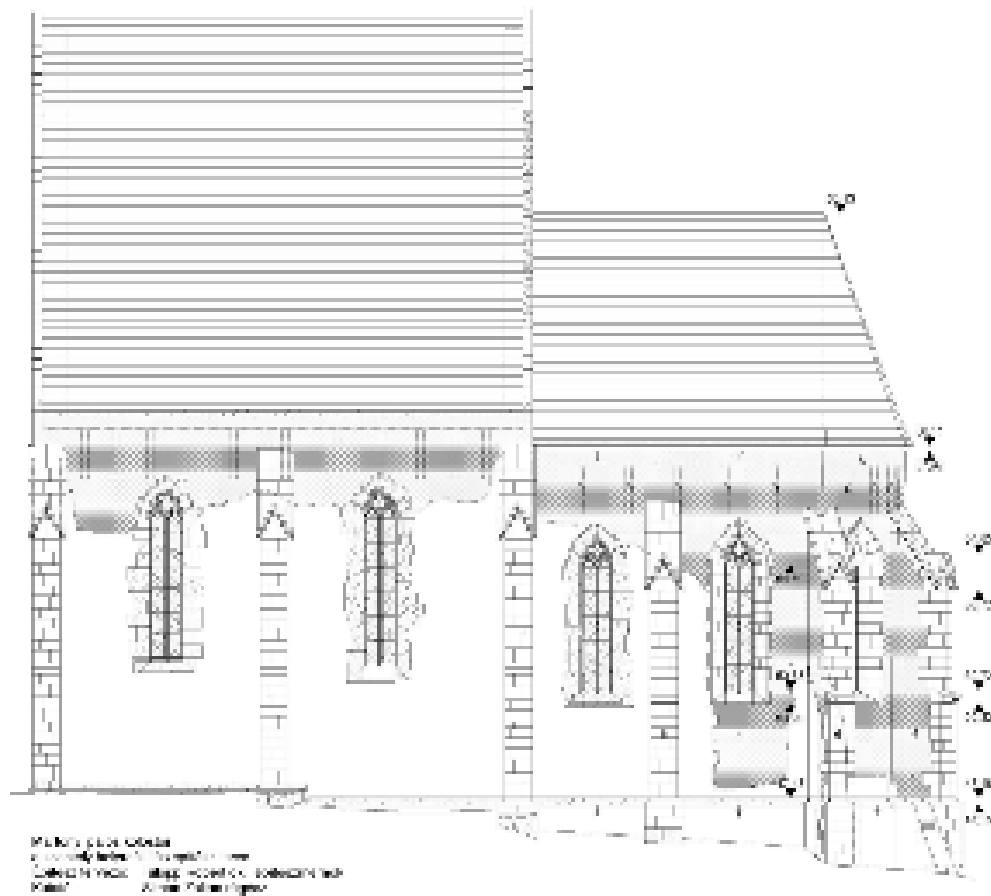
Fülöpp Róbert szentély rekonstrukciós terve
